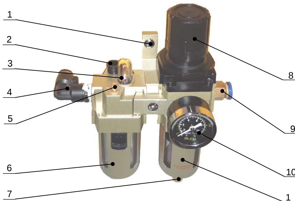
Рис. 2. Система воздухоподготовки
